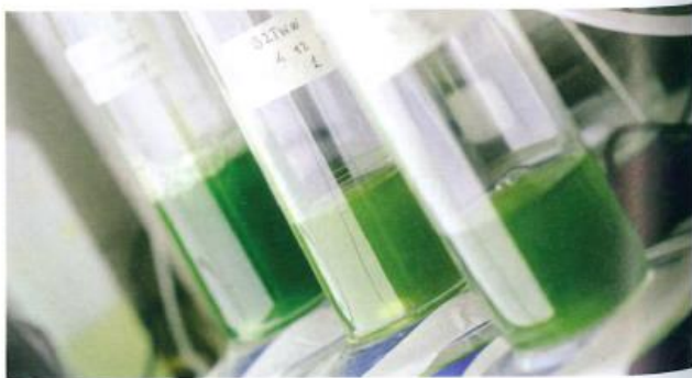
Coltivazioni di laboratorio di microalghe
