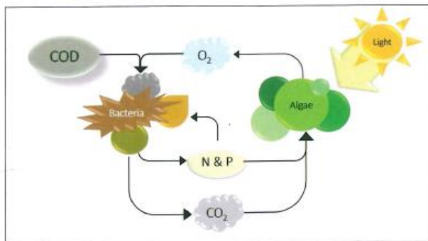
Schema esemplificativo delle interazioni alghe e batteri che possono instaurarsi all'interno di acque reflue
